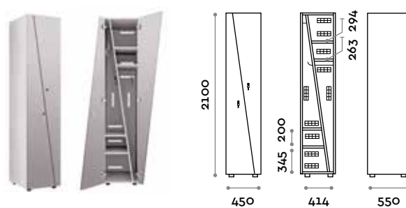
ATRO2-19 Armadio 2 ante trapezoidali
