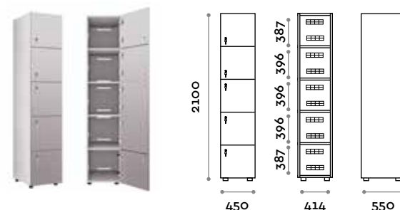
ANB05-19 Armadio 5 ante
