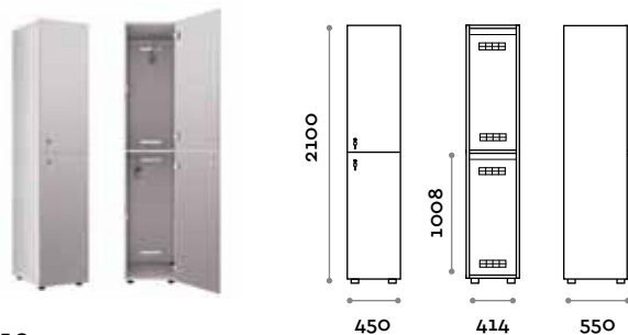
ANBo3-19 Schränk mit 2 „L“-förmigen Türen
