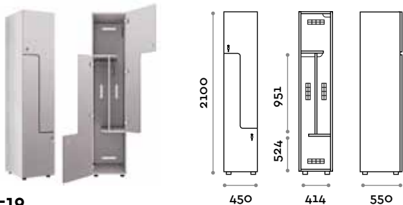
ATRo2-19 Schränk mit 2 trapezförmigen Türen
