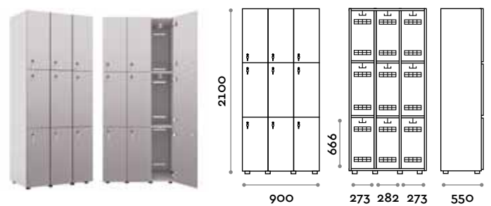
ANB93-19 Armario tres cuerpos 9 hojas con gancho
