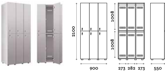
ANB90-19 Casier triple 6 portes
