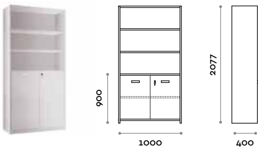
MA100 Meuble avec compartiment et portes
