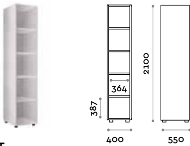
ACCDRT Meuble pour serviettes sale/propre avec 1 porte, 2 tablettes fixes et trappe en aluminium pour le bac à linge
