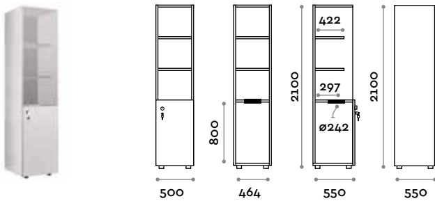
MA100 Meuble avec compartiment et portes
