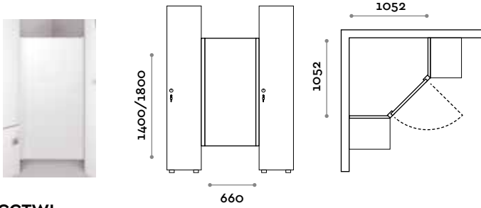
ACCTWL Armario para toallas abierto con 4 repisas
