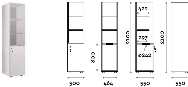
MA100 Mueble con receptáculo y hojas
