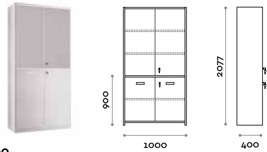
MB100 Meuble à deux portes avec serrure
